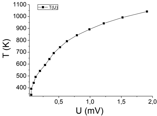
4. sz. ábra. A hőmérséklet függése a feszültségtől
