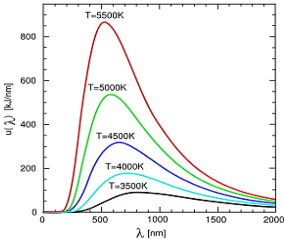
1.sz. ábra. A hőmérsékleti sugárzás a hullámhossz függvényében. A görbék maximumához tartozó hullámhossz a hőmérséklet növekedésével balra tolódik
