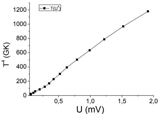
5. sz. ábra. A hőmérséklet negyedik hatványának függése a feszültségtől
