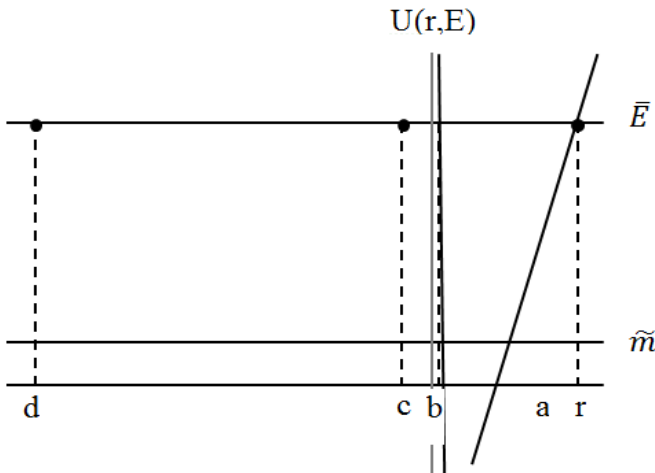
2. ábra. Effektív potenciál az (1) egyenletrendszerre a (10) potenciáltól, ha \lambda < \frac{1}{2}, \sigma > 0 ; a, b, c és d - a (7) kvázi impulzus gyökei.
