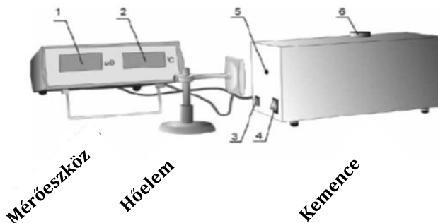
3. sz. ábra. A mérőberendezés felépítése
